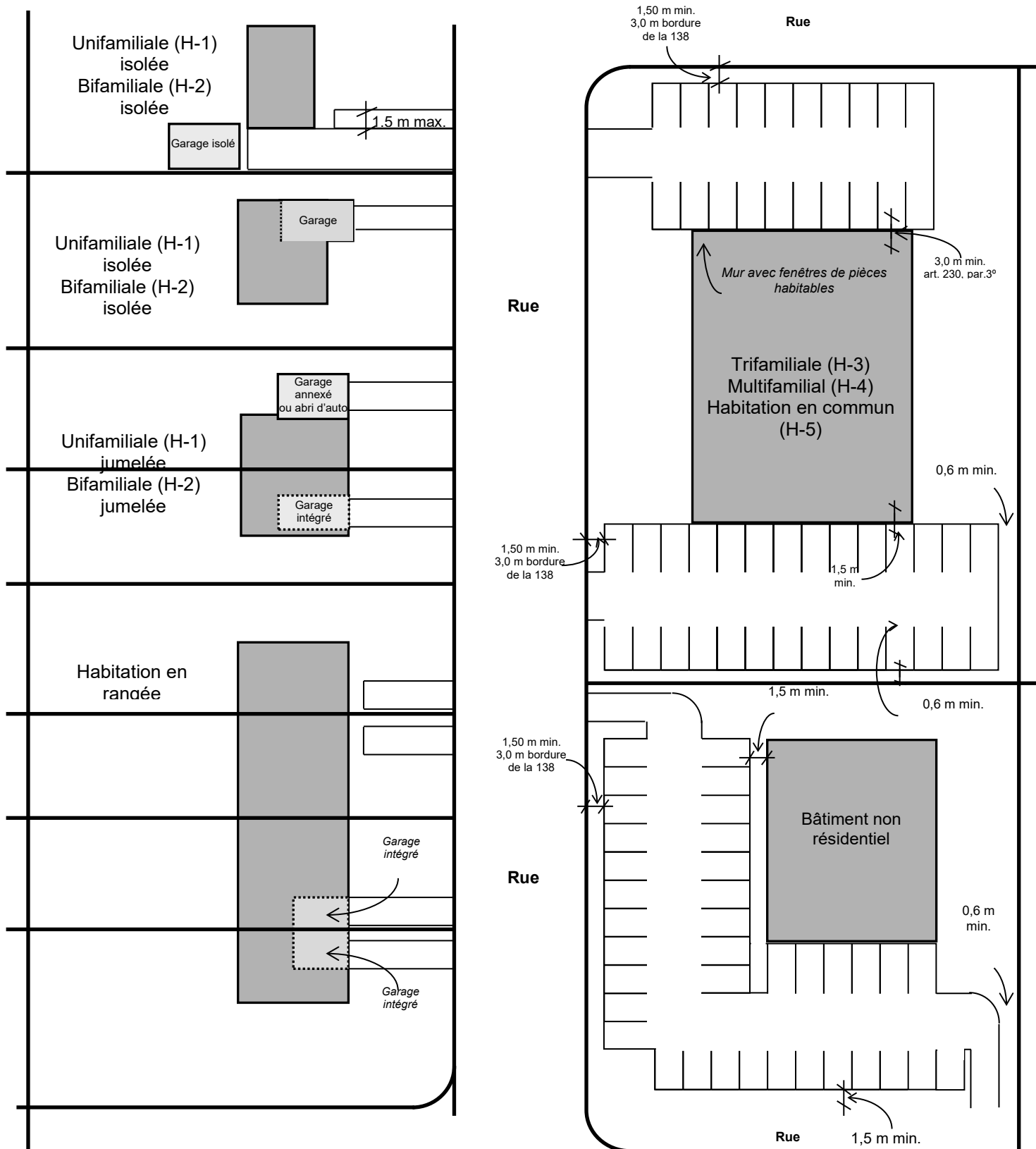
FIGURE 29 Localisation d'une aire de stationnement
