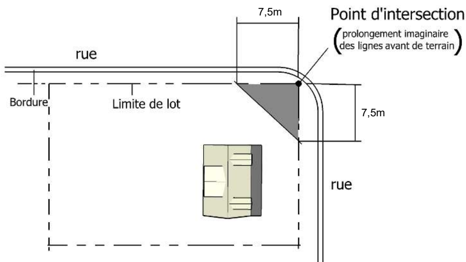
FIGURE 32 Triangle de visibilité
