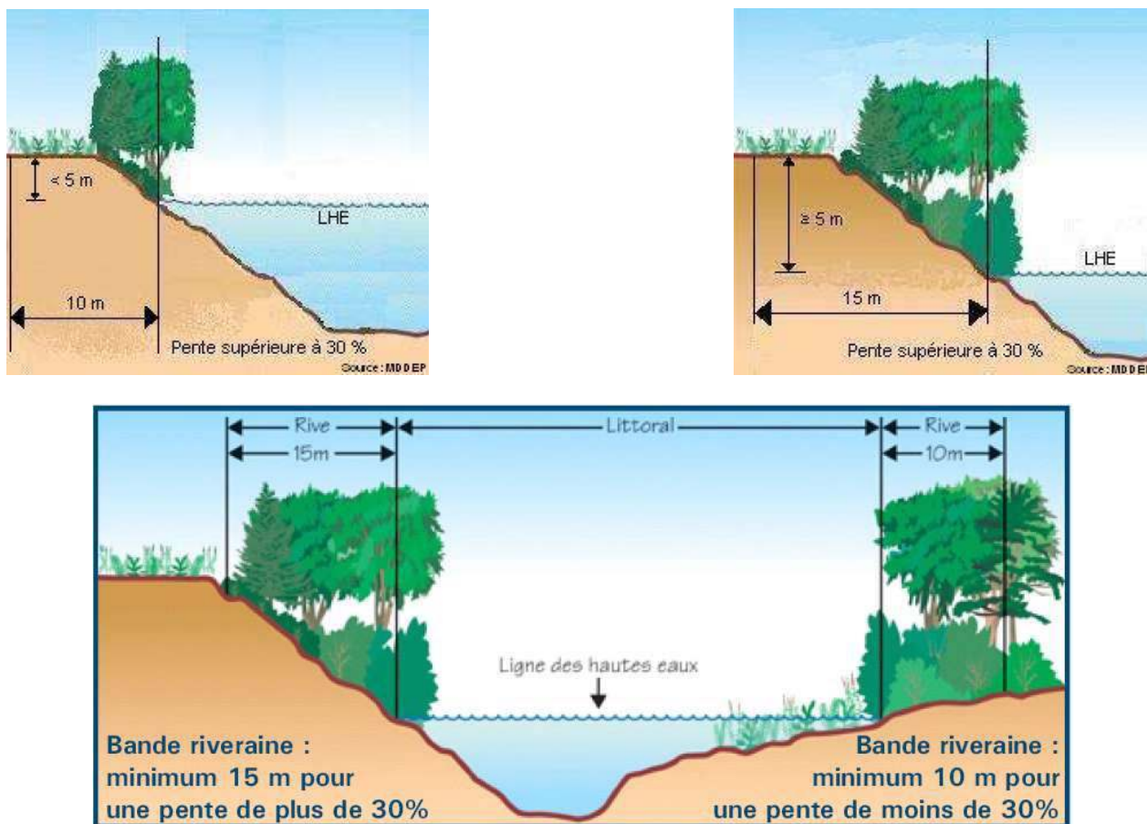
FIGURE 40 Largeur de la rive
