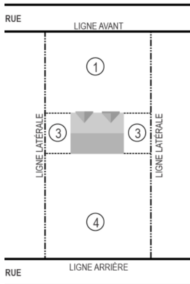
SCHÉMA G Terrain intérieur - 2
