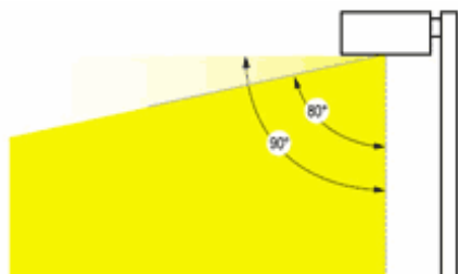
FIGURE 23 Luminaire à défilement absolu
